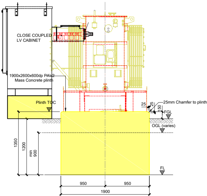
Section 01
