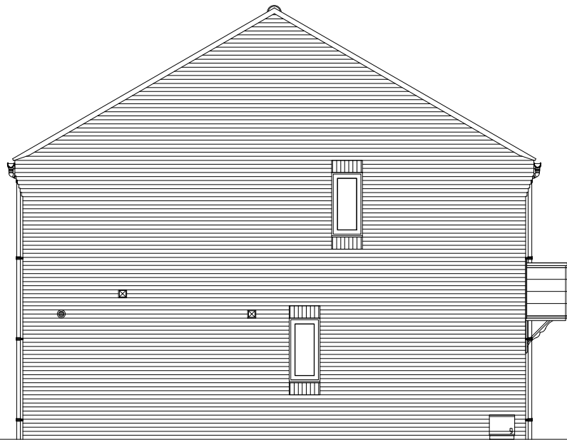
END ELEVATION
