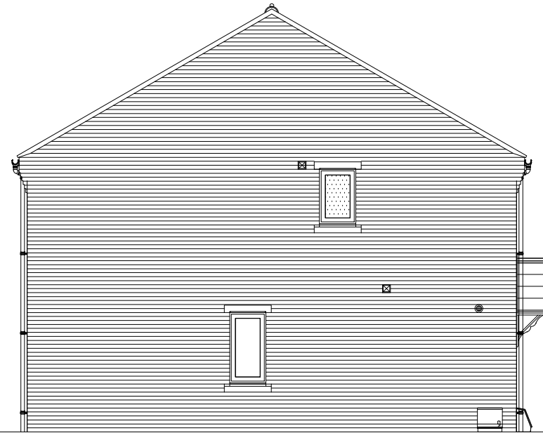
END ELEVATION
