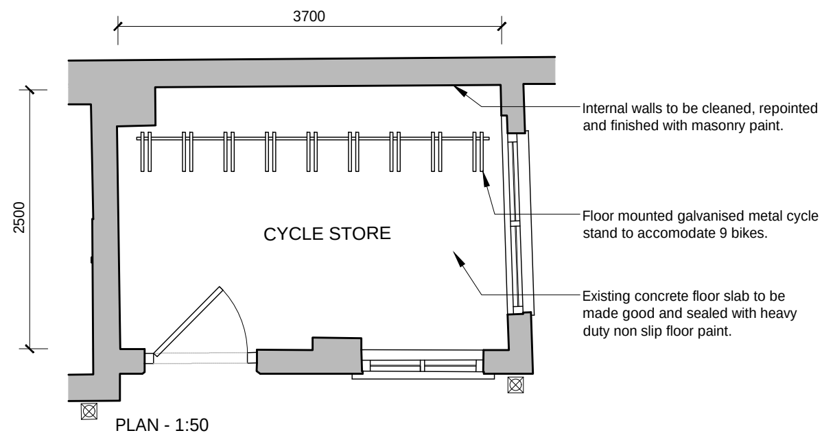
PLAN - 1:50
