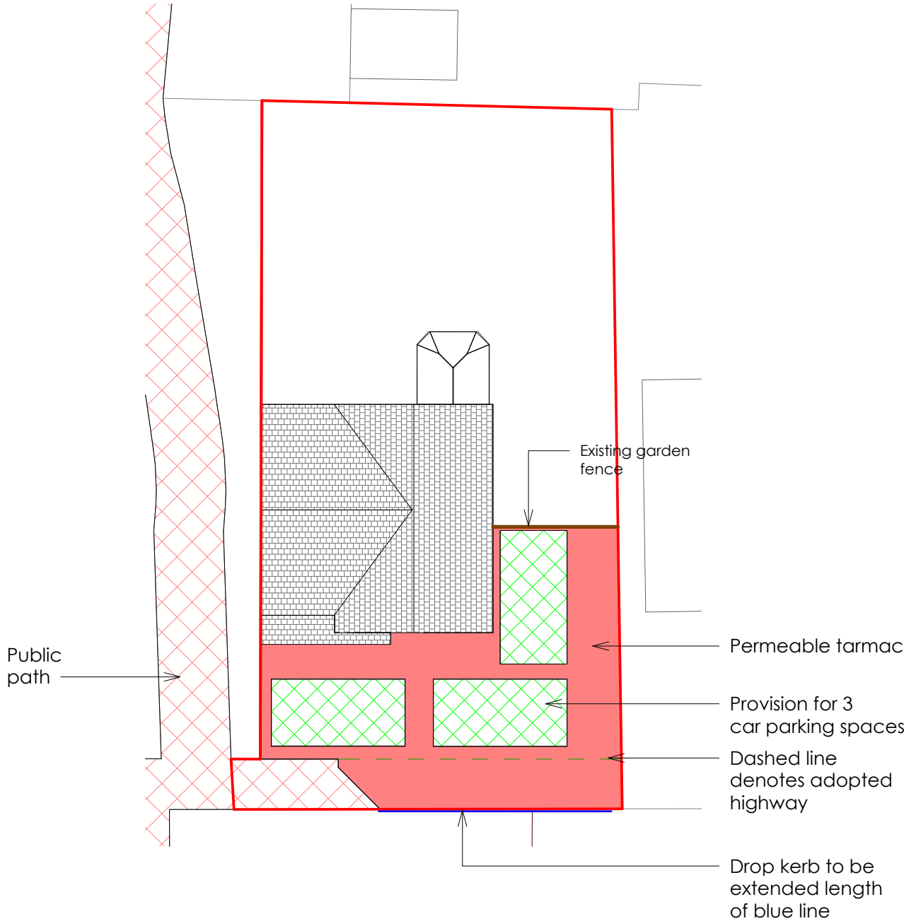
Site Plan 1 : 200
