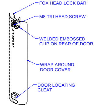
DOOR DETAIL
