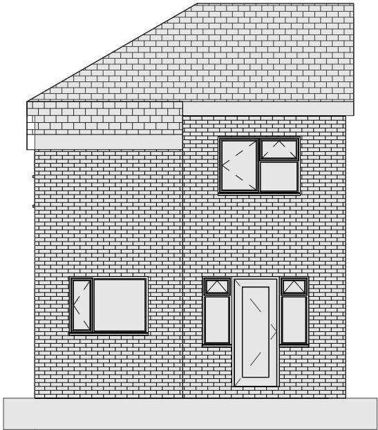
2 Existing Rear SCALE: 1 : 100
