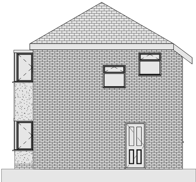
4 Existing East SCALE: 1 : 100
