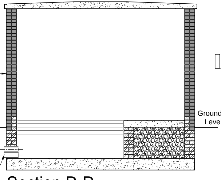
Section D-D
