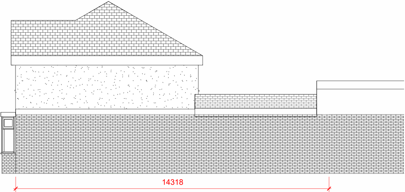
East 1 : 100
