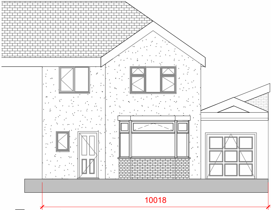
Front 1 : 100
