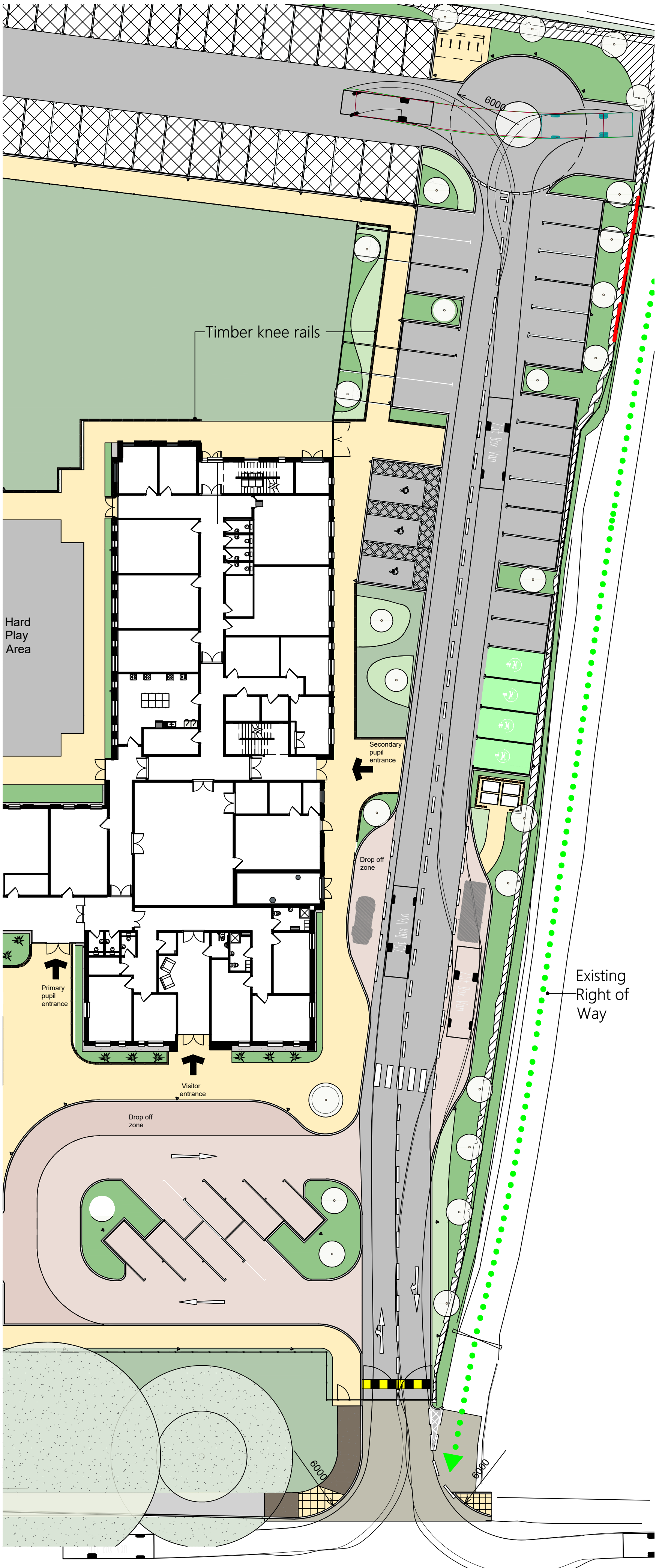
7.5t Box Van - Layby and Turning Head
