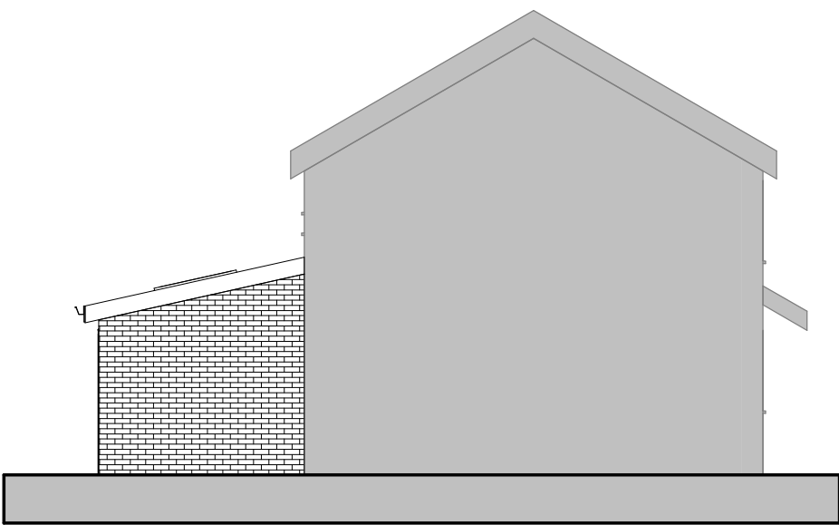
West 1 : 100
