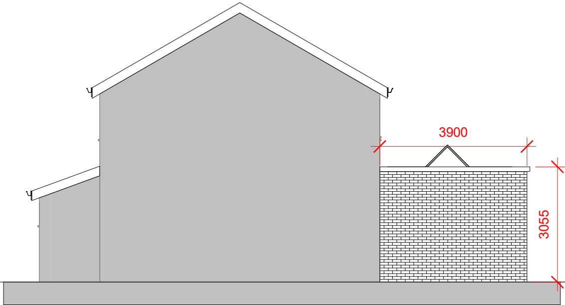
East 1 : 100
